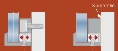
SCHRAUBMONTAGE auf Beton oder Holz
